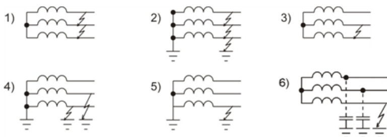
Rys.1. Rodzaje zwarc: 1) fazowe; 2) 3-fazowe z ziemią; 3) dwufazowe; 4) dwufazowe z ziemią; 5) 1-fazowe z punktem neutralnym uziemionym; 6) 1-fazowe w sieciach z punktem neutralnym izolowanym
