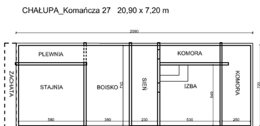
Rys. 2. Plan chałupy łemkowskiej z miejscowości Komańcza, opracowanie A. Mikrut na podstawie karty ewidencyjnej obiektu
