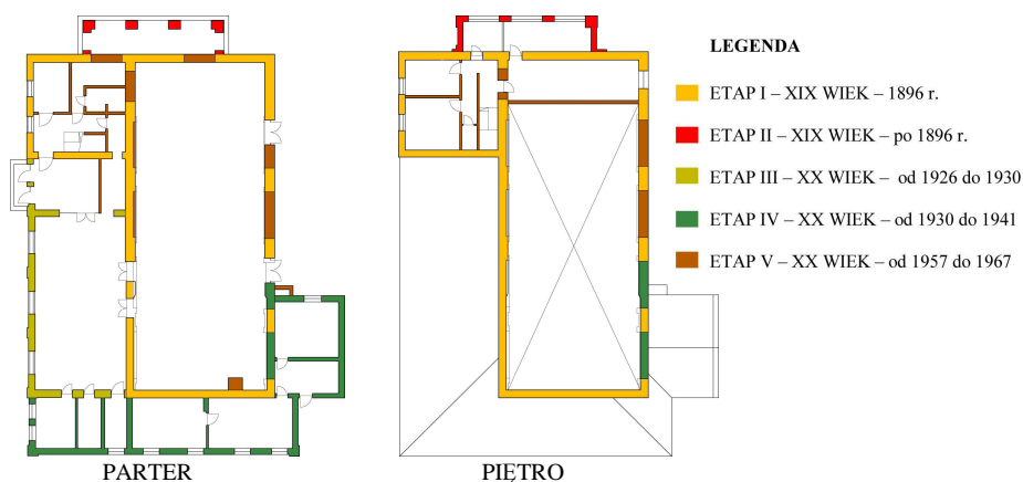
Ryc.1. Schemat stratygrafii gmachu Towarzystwa Gimnastycznego „Sokół” w Łańcutie (autor: T. Huk na podstawie „Analizy historycznej z badaniami architektonicznymi” 4 )
